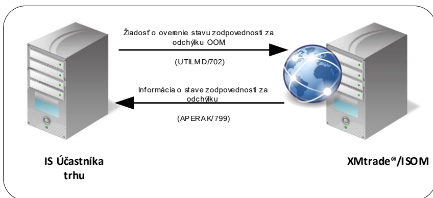
Obrázok 36 Rozhranie pre overenie zabezpečenia zodpovednosti za odchýlku
