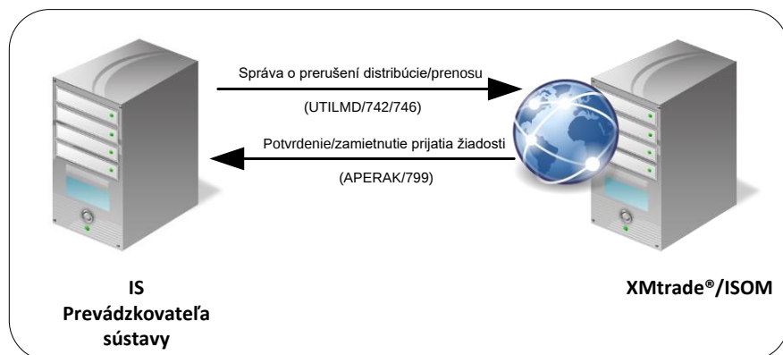
Obrázok 10 Rozhranie pre správu o prerušení distribúcie/prenosu
