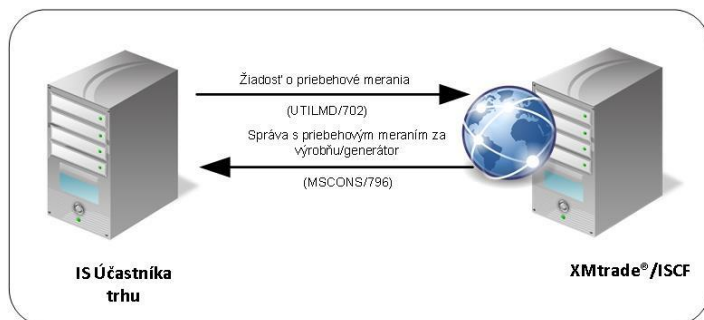
Obrázok 19 Rozhranie pre žiadosť o priebehové merania výrobní/generátora
