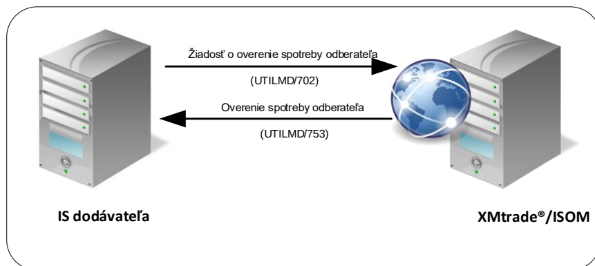
Obrázok 32 Rozhranie pre overenie spotreby odberateľa
