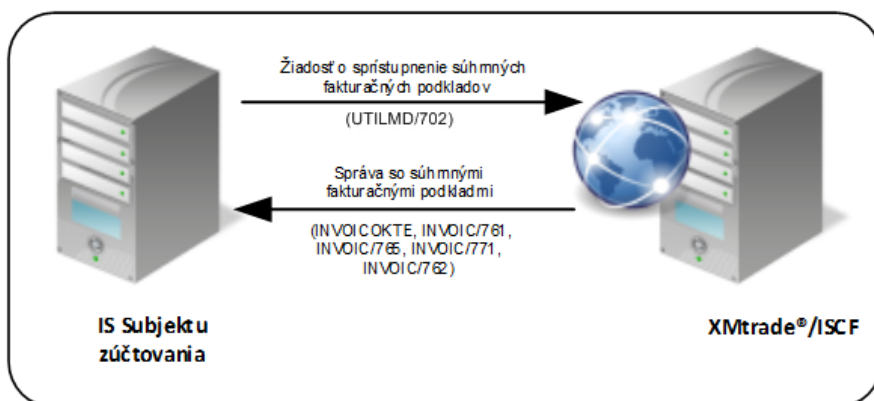
Obrázok 26 Rozhranie pre žiadosť o súhrnné fakturačné podklady
