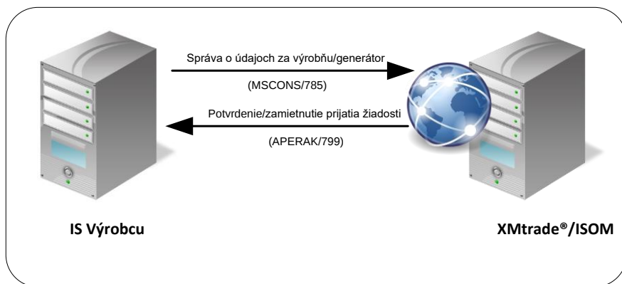
Obrázok 16 Rozhranie pre správu o údajoch za výrobu/generátor
