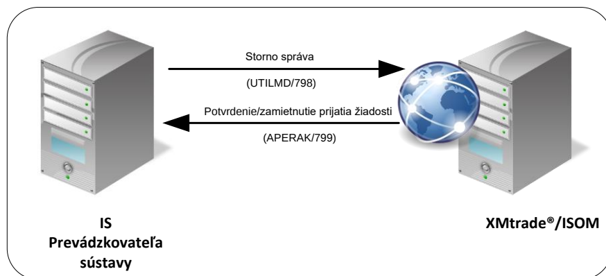
Obrázok 7 Rozhranie pre storno správu
