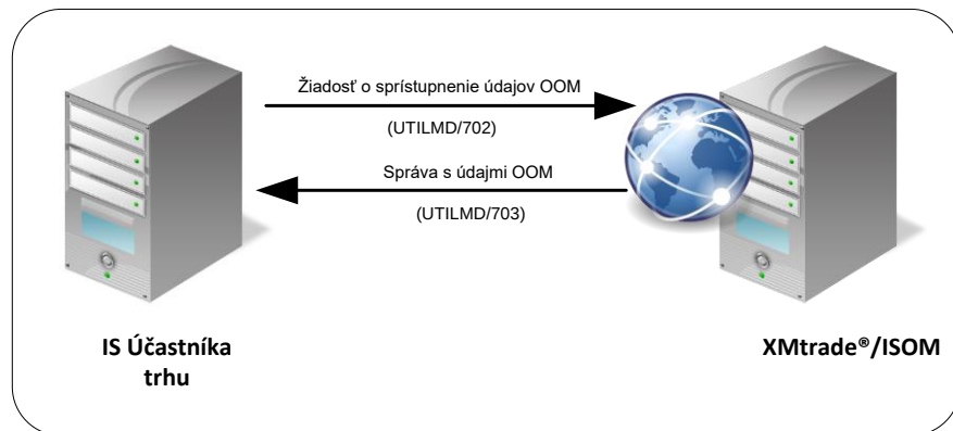
Obrázok 4 Rozhranie pre žiadosť o sprístupnenie údajov OOM
