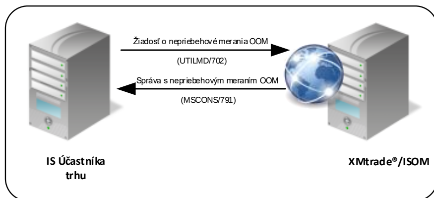
Obrázok 15 Rozhranie pre žiadosť o nepriebegové merania OOM
