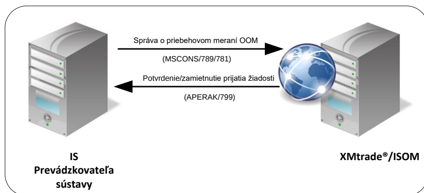
Obrázok 12 Rozhranie pre správu o priebehovom meraní OOM
