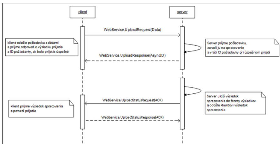
Obrázok 2 Princíp asynchrónnej komunikácie
