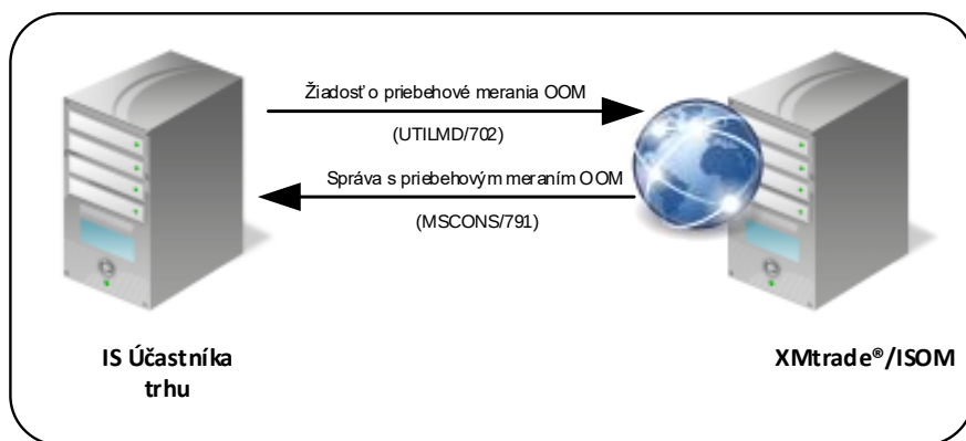
Obrázok 13 Rozhranie pre žiadosť o priebehové merania OOM
