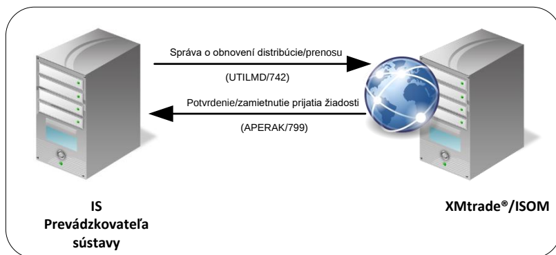
Obrázok 11 Rozhranie pre správu o obnovení distribúcie/prenosu
