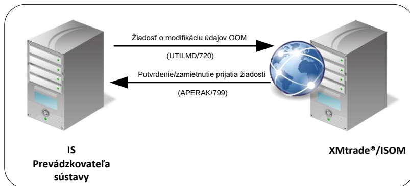
Obrázok 5 Rozhranie pre žiadosť o modifikáciu údajov OOM
