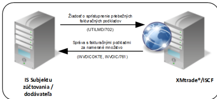
Obrázok 25 Rozhranie pre žiadosť o priebežné fakturačné podklady
