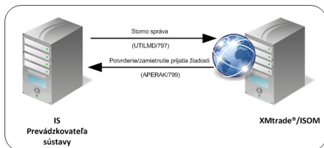
Obrázok 20 Rozhranie pre storno správu
