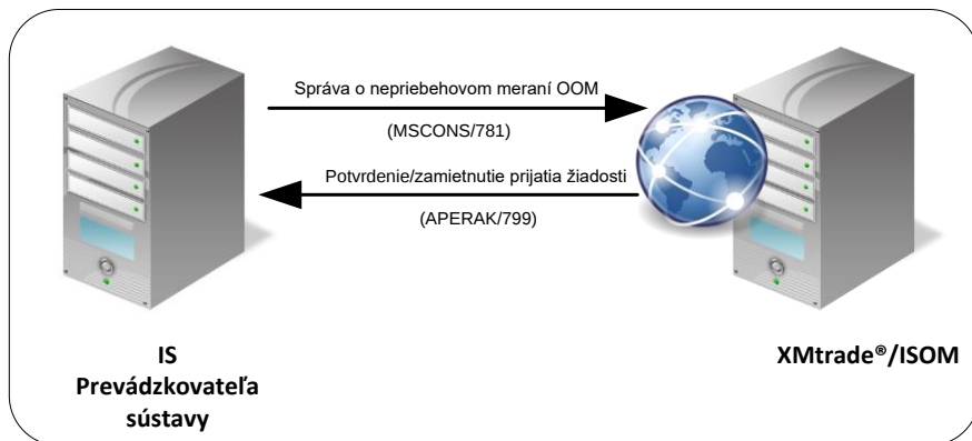
Obrázok 14 Rozhranie pre správu o nepribehovom meraní OOM
