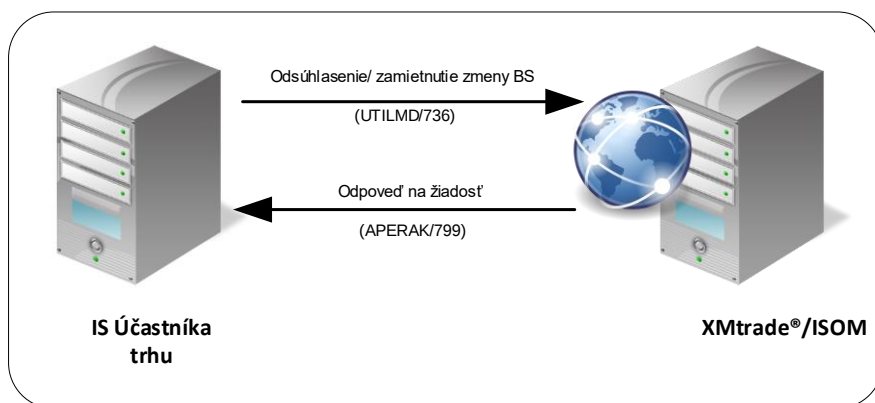
Obrázok 34 Rozhranie pre zamietnutie zmeny BS
