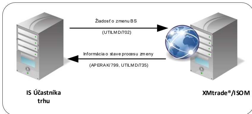
Obrázok 33 Rozhranie pre žiadosť o zmenu bilančnej skupiny
