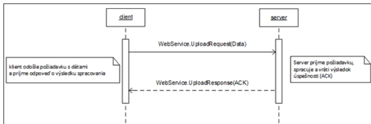
Obrázok 1 Princíp synchronnej komunikácie
