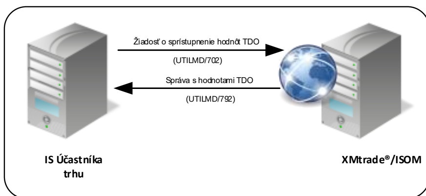
Obrázok 23 Rozhranie pre žiadosť o sprístupnenie hodnôt TDO
