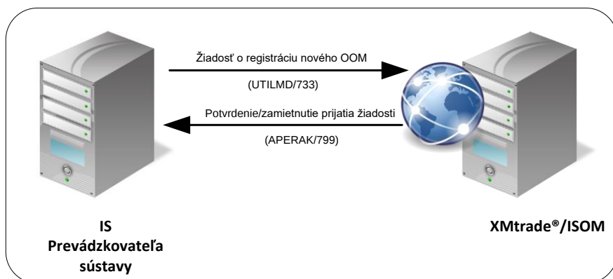
Obrázok 3 Rozhranie pre žiadosť o registráciu nového OOM
