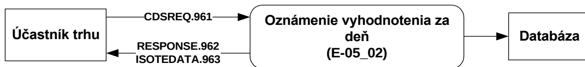
Obrázok 25 Obrázok 28 Schéma oznámenia vyhodnotení DT za deň pre ÚT
