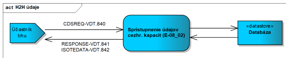
Obrázok 25 Schéma príjmu údajov cezhr. kapacít
