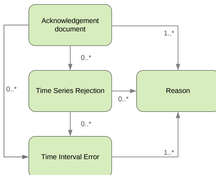
Obrázok 36 Obrázok 39 Schéma štruktúry Acknowledgement
