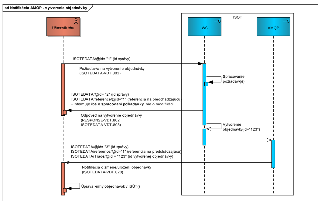
Obrázok 29 Obrázok 32 Schéma posielaných správ – vytvorenie objednávky (AMQP notifikácia)
