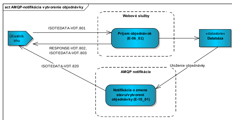
Obrázok 29 Obrázok 32 Schéma posielaných správ – vytvorenie objednávky (AMQP notifikácia)
