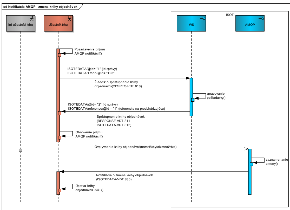
Obrázok 34 Obrázok 37 Schéma následnosti posielaných správ – zmena knihy objednávok (AMQP notifikácia)
