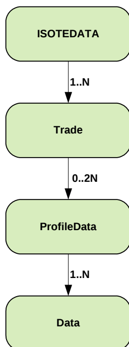
Obrázok 12 Schéma štruktúry objednávky ISOTEDATA-VDT
