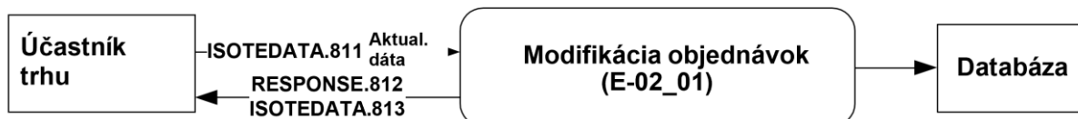
Obrázok 17Obrázok 19 Schéma odstránenia modifikácie objednávky ÚT
