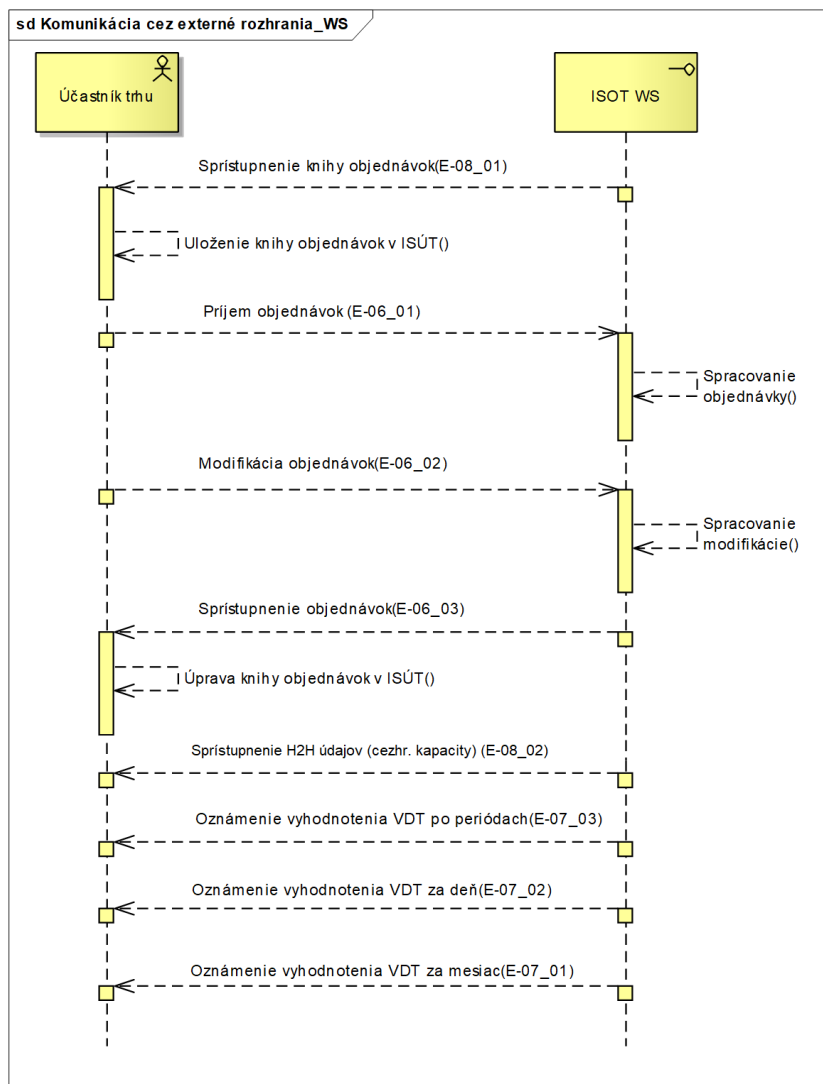
Obrázok 5 Komunikačný scenár webových služieb v režime koordinovaného organizovania vnútrodného trhu
