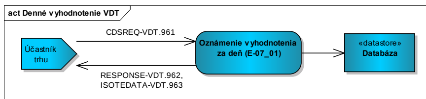
Obrázok 26 Obrázok 29 Schéma oznámenia vyhodnotení VDT za deň pre ÚT
