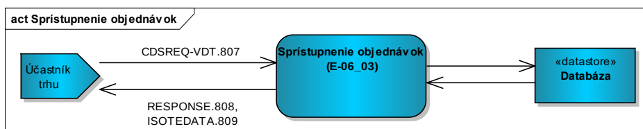
Obrázok 21 Obrázok 23 Schéma príjmu sprístupnenia objednávky ÚT
