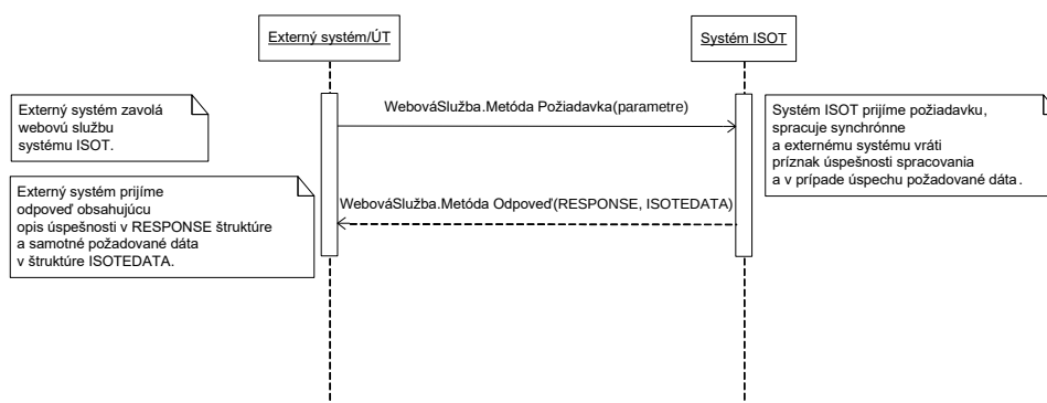
Obrázok 5 Obrázok 7 Princíp synchrónnej komunikácie
