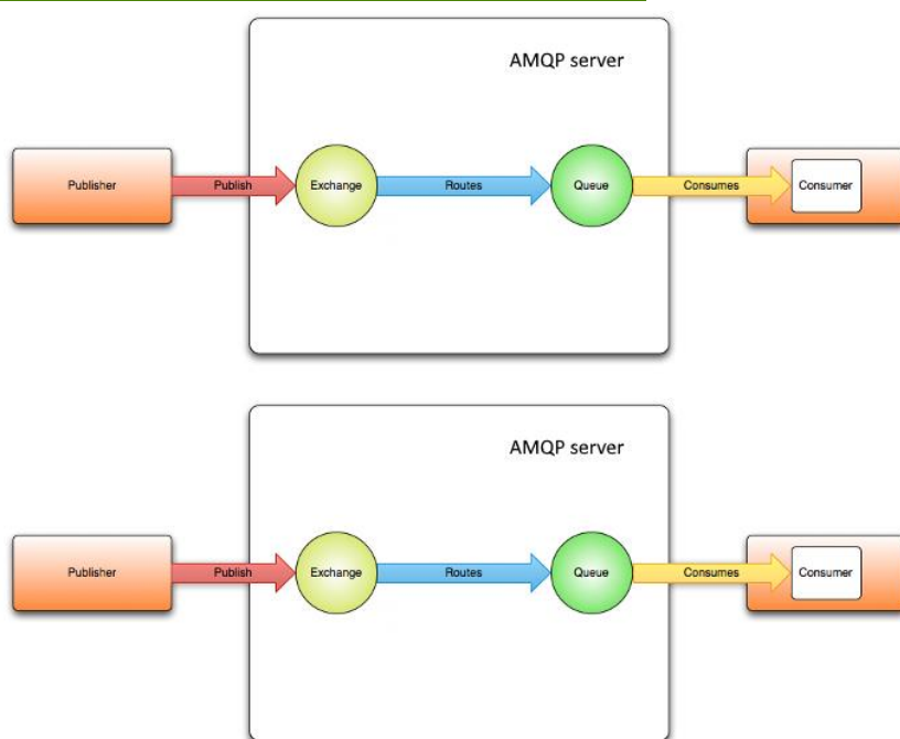
Obrázok 8 Obrázok 9 Koncept AMQP komunikácie
