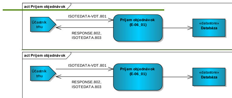
Obrázok 24 Schéma príjmu objednávky ÚT
