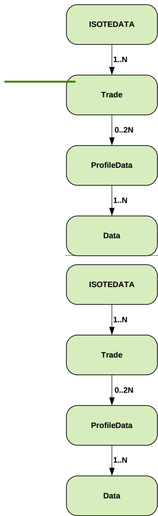
Obrázok 15 Schéma štruktúry ISOTEDATA-VDT
