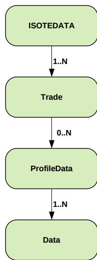
Obrázok 14 Schéma štruktúry výsledkov VDA
