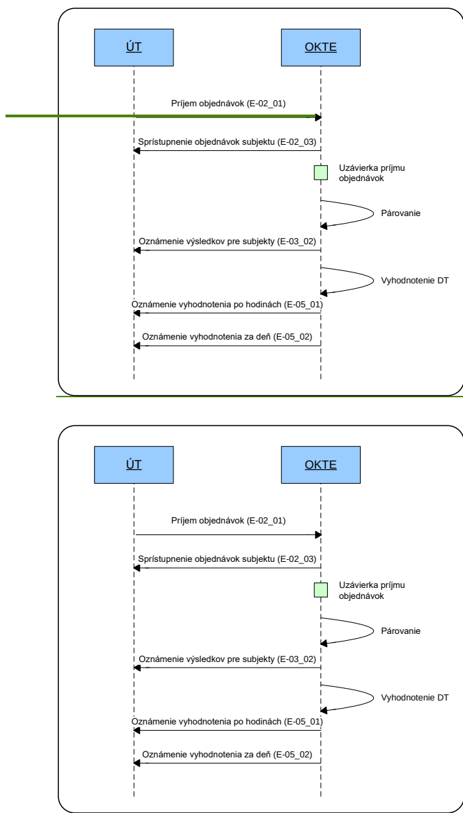
Obrázok 1 Komunikačný scenár v režime organizovania domáceho denného trhu
