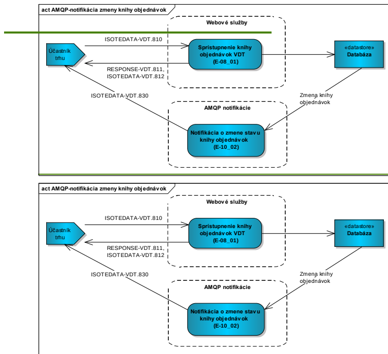
Obrázok 36 Obrázok 43 Schéma posielaných správ – vytvorenie objednávky (AMQP notifikácia)
