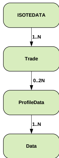
Obrázok 13 Schéma štruktúry objednávky VDA
