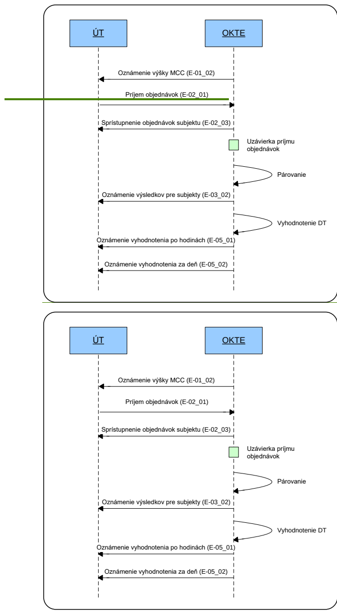
Obrázok 2 Komunikačný scenár v režime koordinovaného organizovania denného trhu
