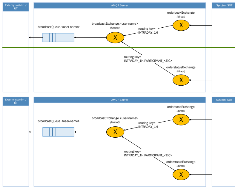
Obrázok 9Obrázok 10 Schéma toku notificačných správ na vnútrodennom trhu
