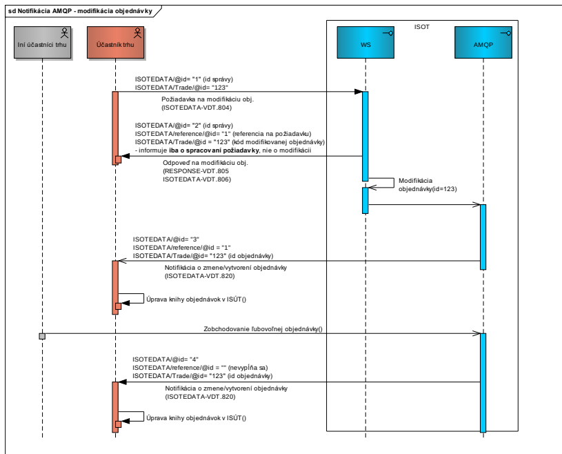
Obrázok 35Obrázok 42 Schéma následnosti posielaných správ – modifikácia objednávky (AMQP notifikácia)
