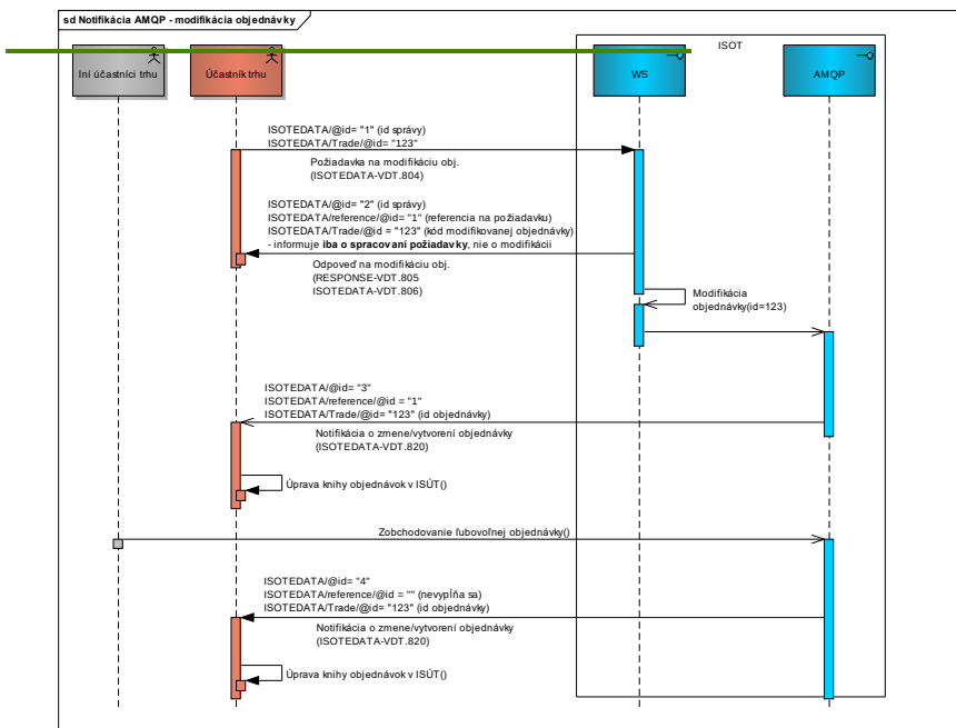
Obrázok 34 Obrázok 41 Schéma posielaných správ – modifikácia objednávky (AMQP notifikácia)
