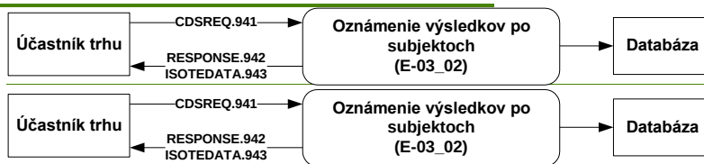
Obrázok 26 Obrázok 33 Schéma oznámenia výsledkov DT po subjektoch pre ÚT
