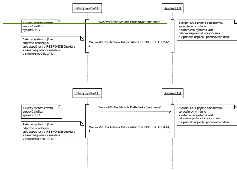
Obrázok 7Obrázok 8 Princíp synchronnej komunikácie
