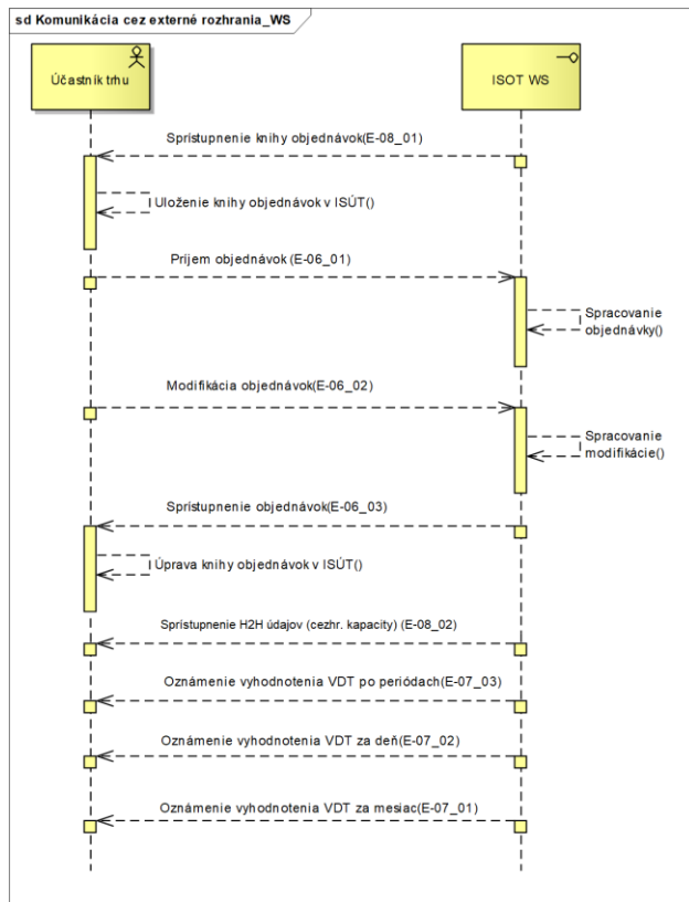
Obrázok 5 Komunikačný scenár webových služieb v režime koordinovaného organizovania vnútrodenného trhu
